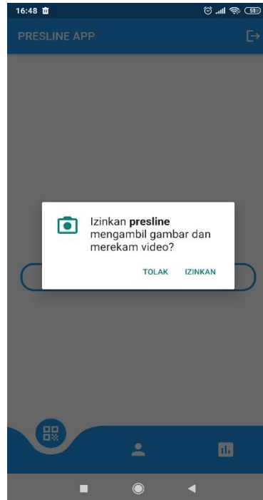
Gambar 5 Perizinan Aplikasi
