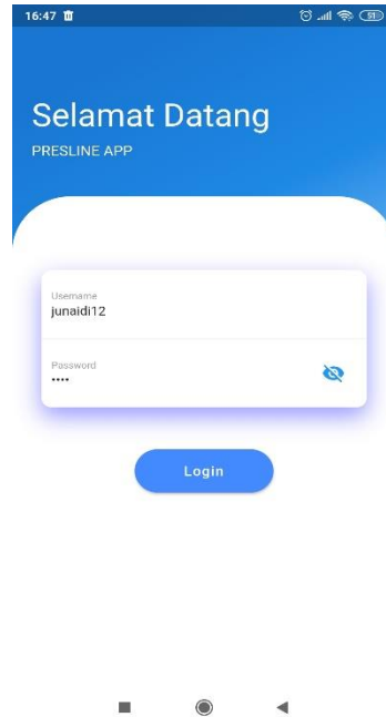
Gambar 3 Menu Login
