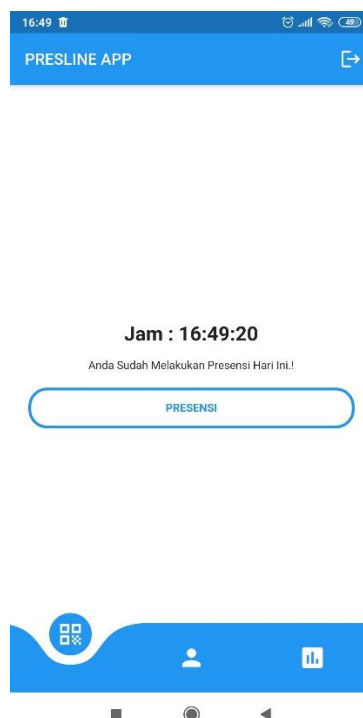
Gambar 8 Presensi Gagal
