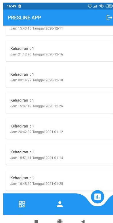
Gambar 10 Menu Kinerja
