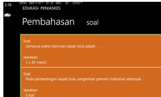
Gambar 5 Tampilan Pembahasan
